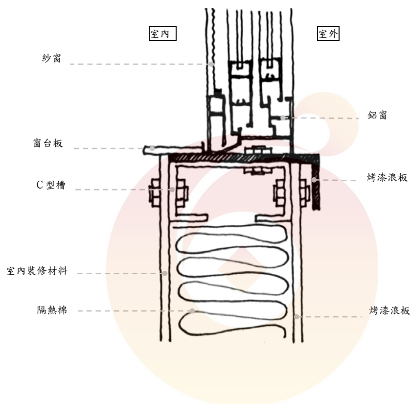
▲窗台縱向剖面圖
