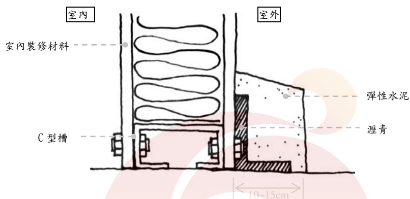
▲ 屋腳縱向剖面
