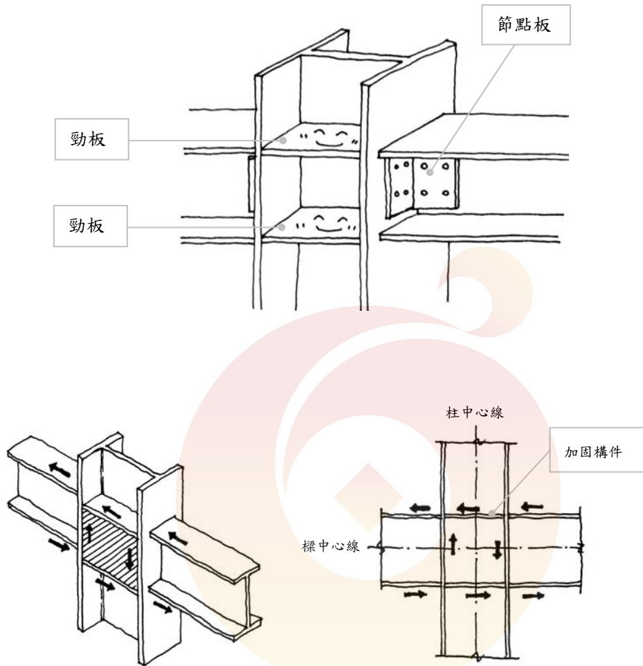
▲水平荷重作用於剪力支承區形成的剪力
